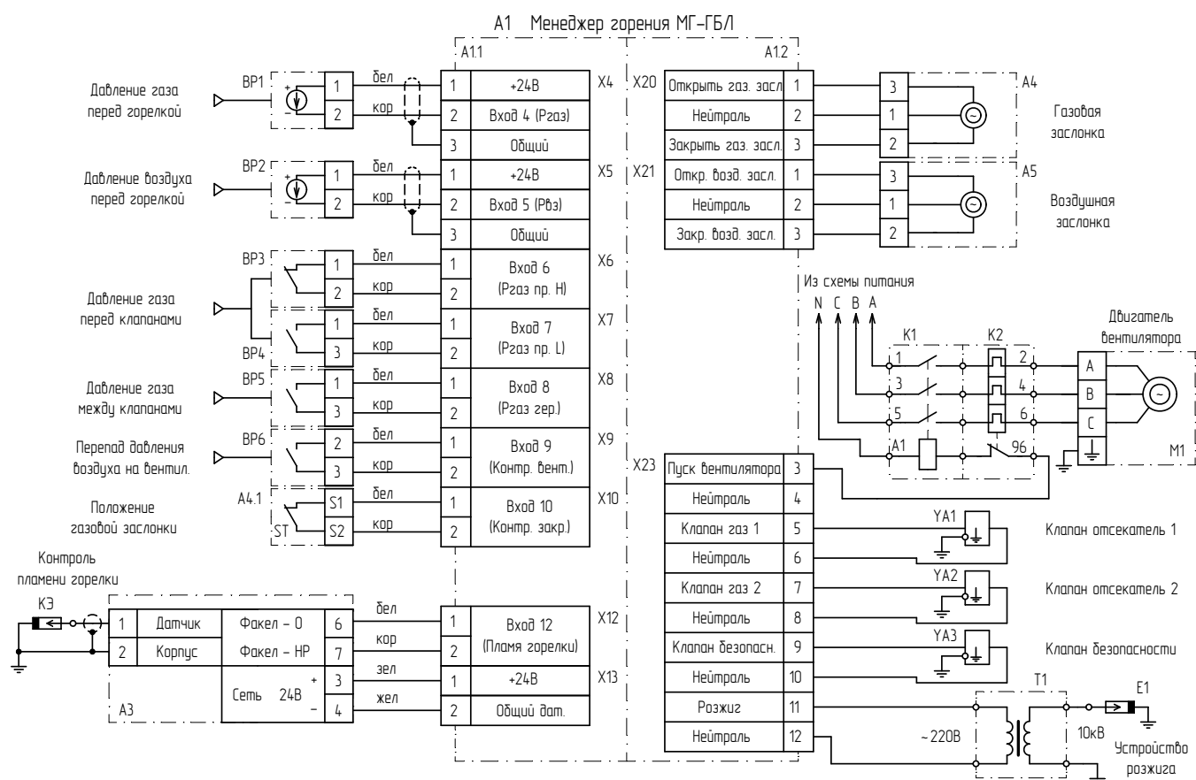
Вариант подключения устройства контроля пламени НП 03-1
