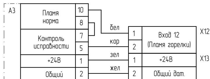
Вариант подключения устройства контроля пламени НП 03-1
