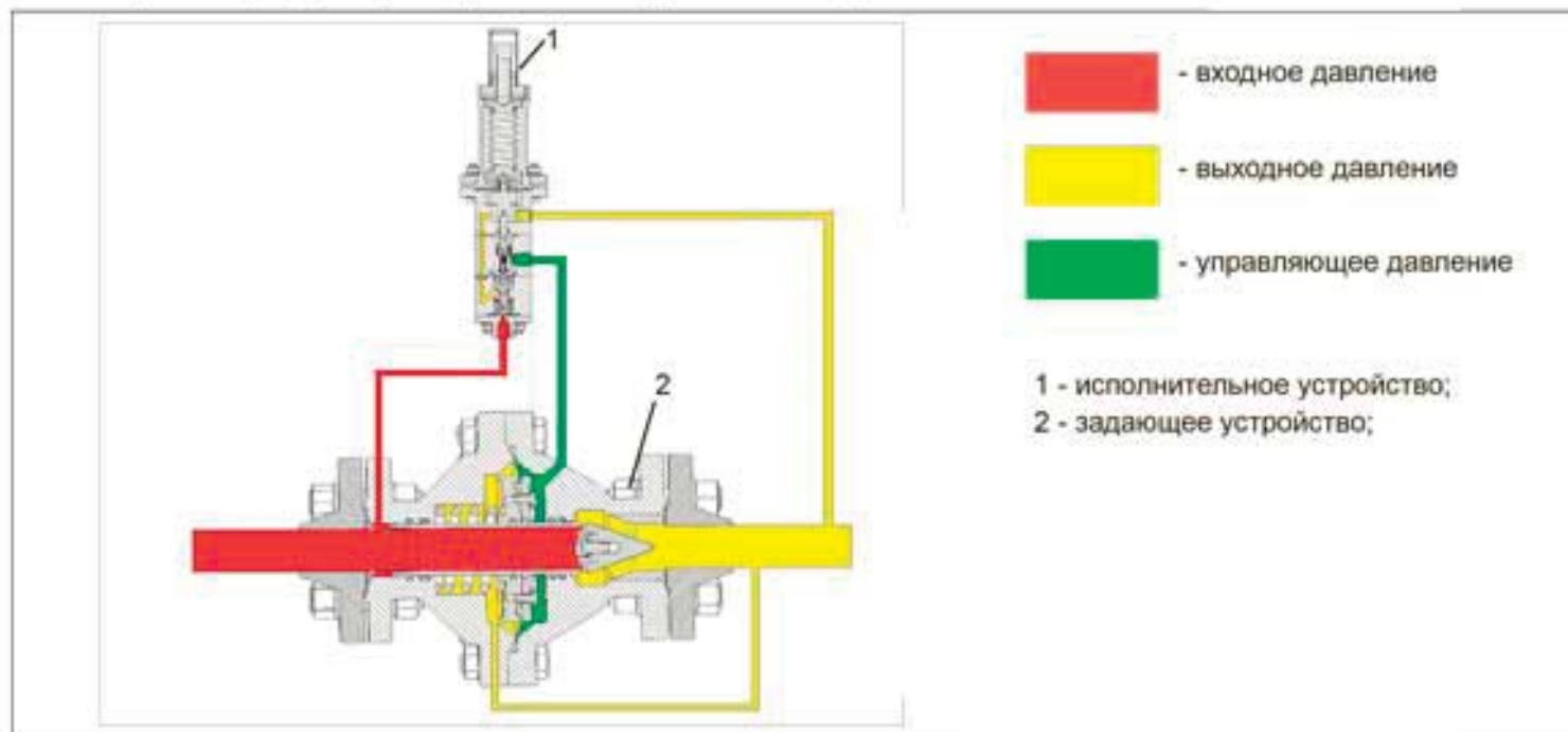
Схема работы регуляторов РДУ-100/50 и РДУ-100/80 с задатчиком ЗУ-3
