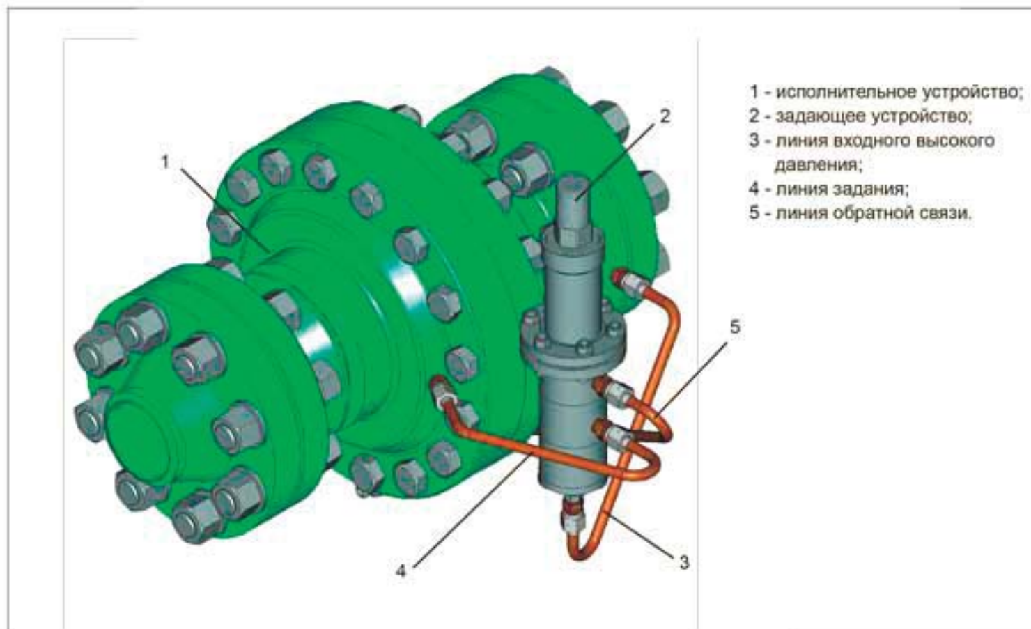
Обвязка регуляторов РДУ-100/50 и РДУ-100/80 задатчиком ЗУ-3
