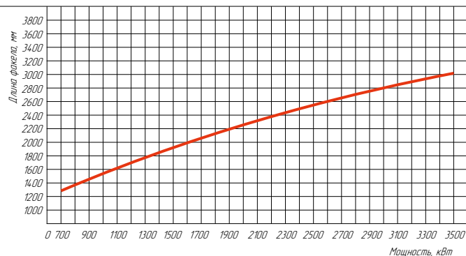
ДЛИНА ФАКЕЛА
