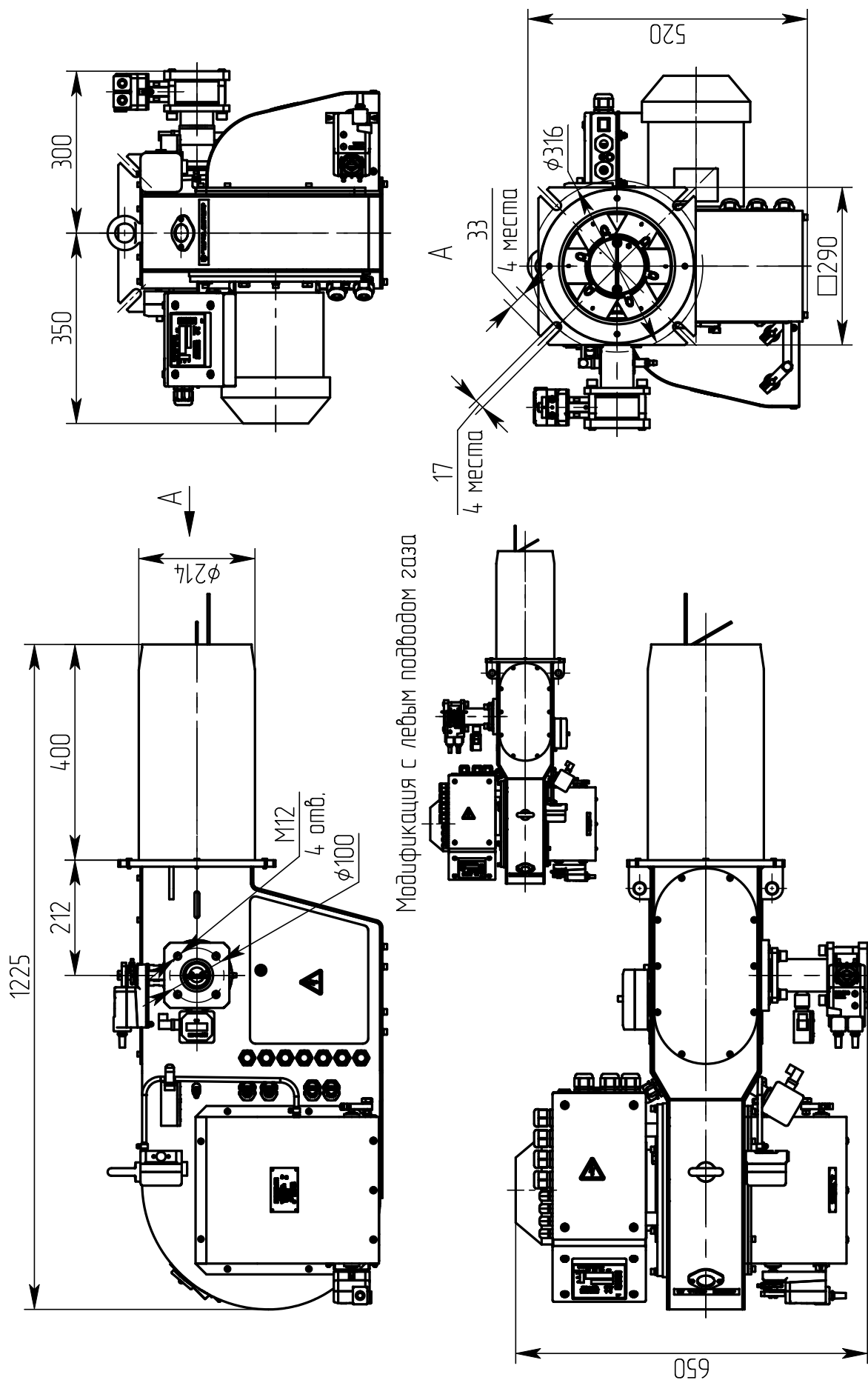
Рисунок А.2. Габаритные и присоединительные размеры горелки
