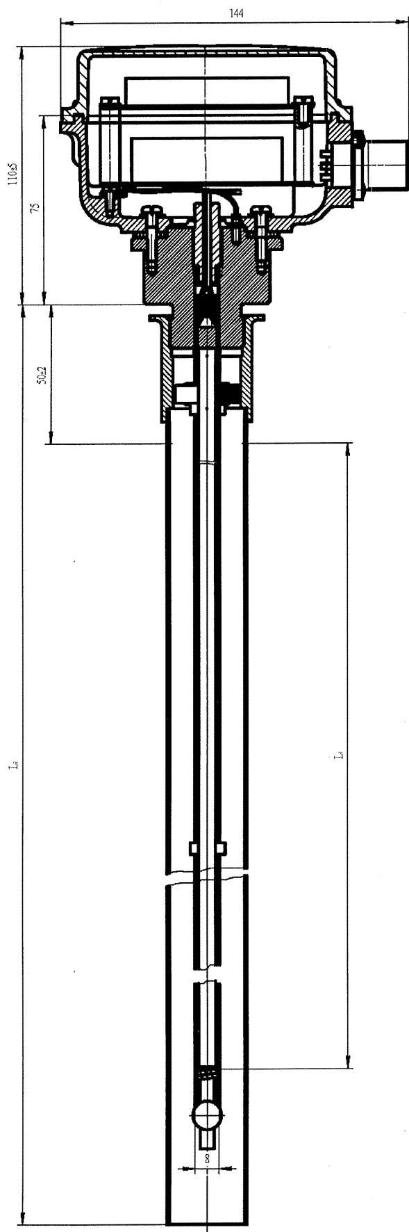
Вариант крепления с прокладкой
