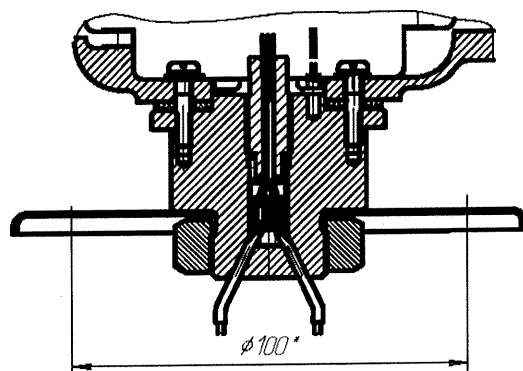
Вариант крепления фланцем
