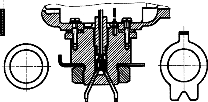
Вариант крепления с прокладкой
